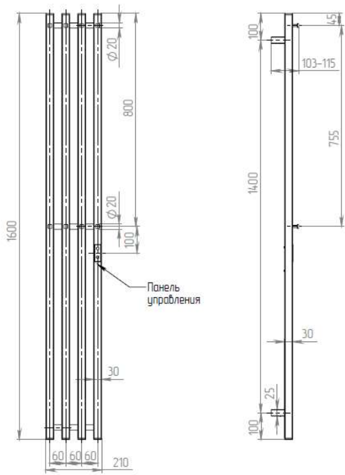
Электрический полотенцесушитель ДВИН Модель X-4 plaza neo -1600x180
